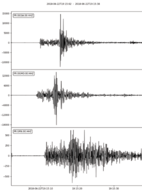
Figure 2: Trois enregistrements des voies verticales des stations OGSA, OGMO, GRN. Temps total des enregistrements 40 secondes.
