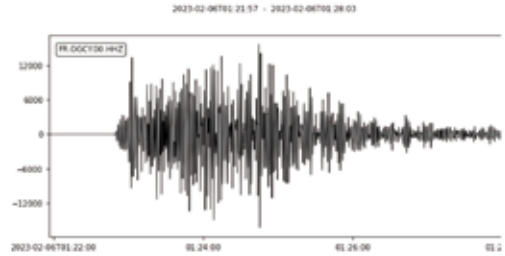
Figure 3: Enregistrement de la voie verticale de la station OGCY le 6 février à 1h20 UTC. Temps total des enregistrements 6 minutes.
