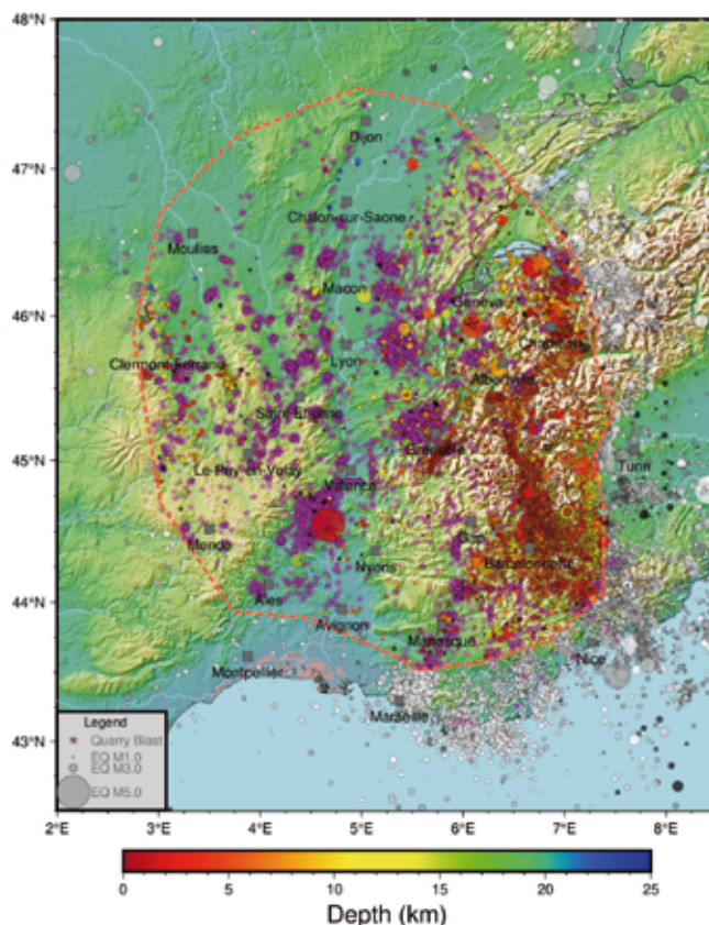
Figure 1: Carte générée depuis le catalogue de sismicité SISMALP, représentant les détections d'événements sismiques de 1987 à 2023, concentrées sur la zone des Alpes (tirets rouges). Les étoiles violettes représentent les tirs de carrière, les cercles représentent les séismes, et leurs tailles et couleurs représentent respectivement leur magnitude et leur profondeur.
